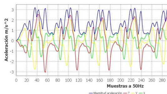
Figura 6: Señales de aceleración muestreadas en una ventana de 8 s, magnitud, X, Y y Z.
